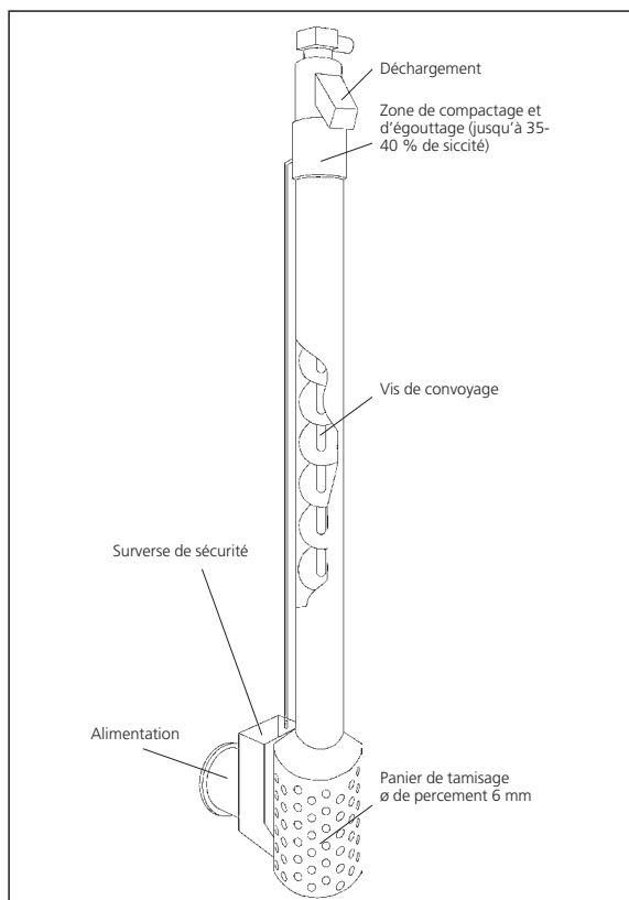
Dans sa version calorifugée, l'unité de tamisage s'installe sans complication en extérieur
